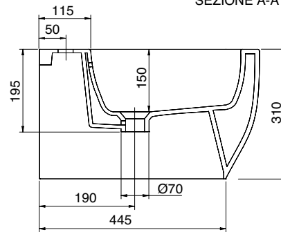
SEZIONE A-A
