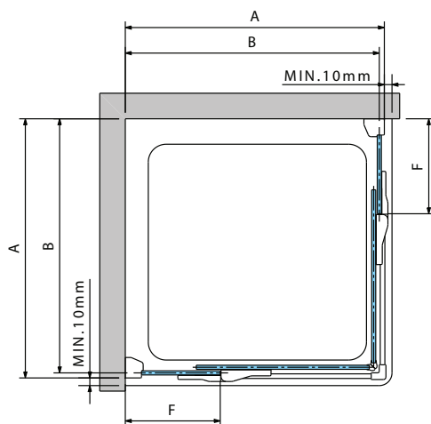
GALA A WERSJA DO MONTAŻU Z PROFEM PRZYŚCIENNYM
