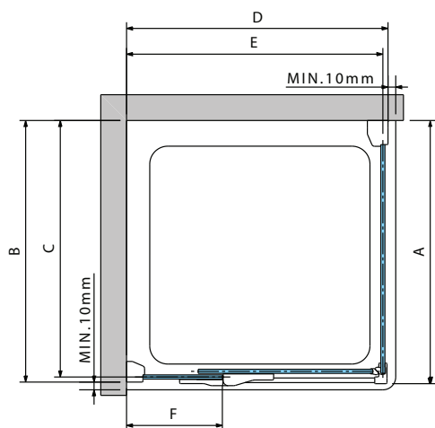
GALA G WERSJA DO MONTAŻU Z PROFEM PRZYŚCIENNYM
