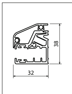
Profil poszerzający
